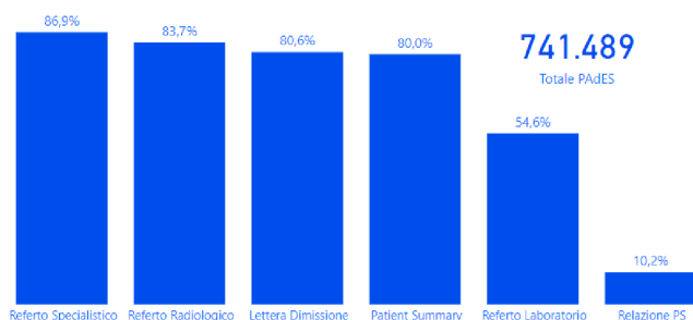
% documenti firmati PAdES per tipologia di documento
