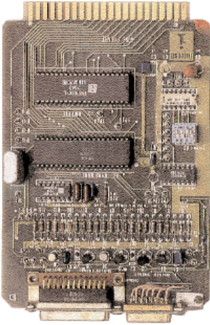
In alto, circuito stampato di un piccolo computer.
